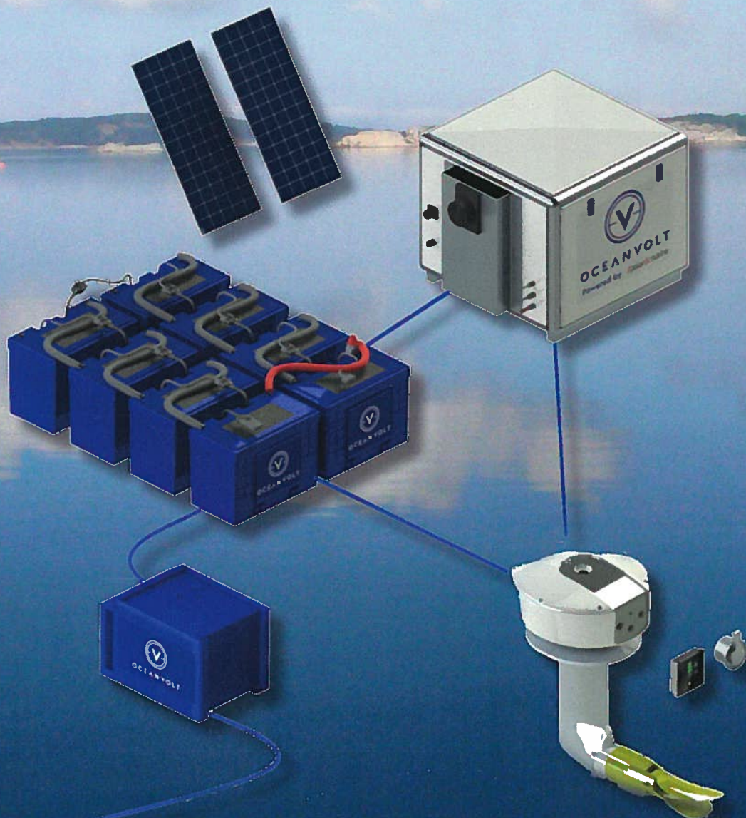
Arcona 380Z (Zero Emission) – komponenter for eldrift
